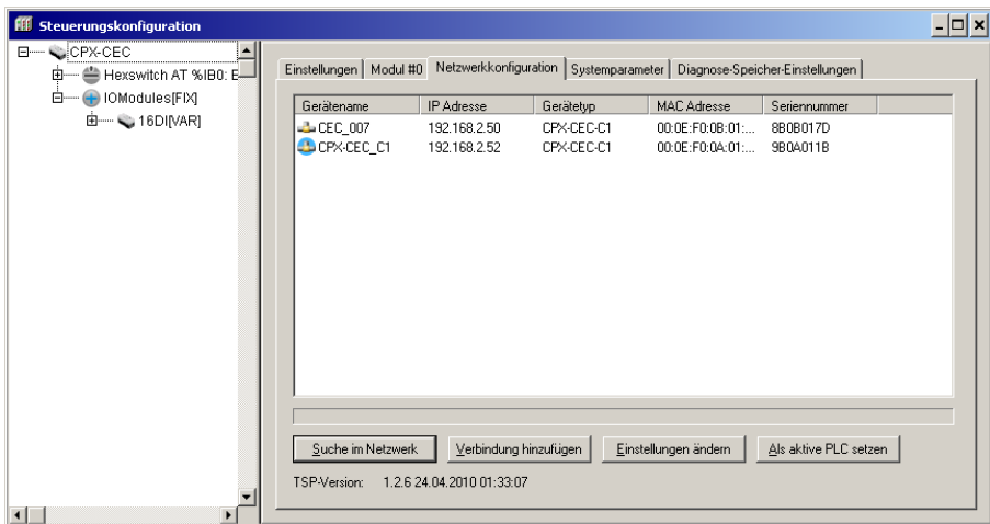
Bild 3/1: Netzwerkconfiguration am Beispiel des CPX-CEC-C1
