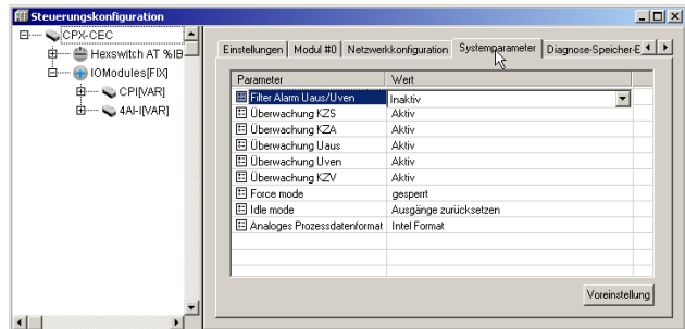
Bild 3/7: Register “Systemparameter”
