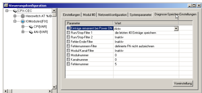
Bild 3/8: Register “Diagnose-Speicher-Einstellungen”
