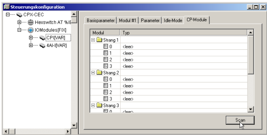
Bild 3/3: Register “CP-Module”
