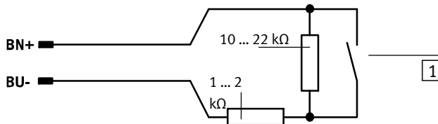
Fig. 14 Anschluss von beschalteten mechanischen Kontakten
