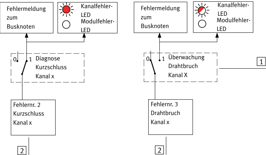
1 Kanalspezifische Modul-Parameter (Schalterstellung zeigt die Voreinstellung) 2 Kanalspezifische Fehler
