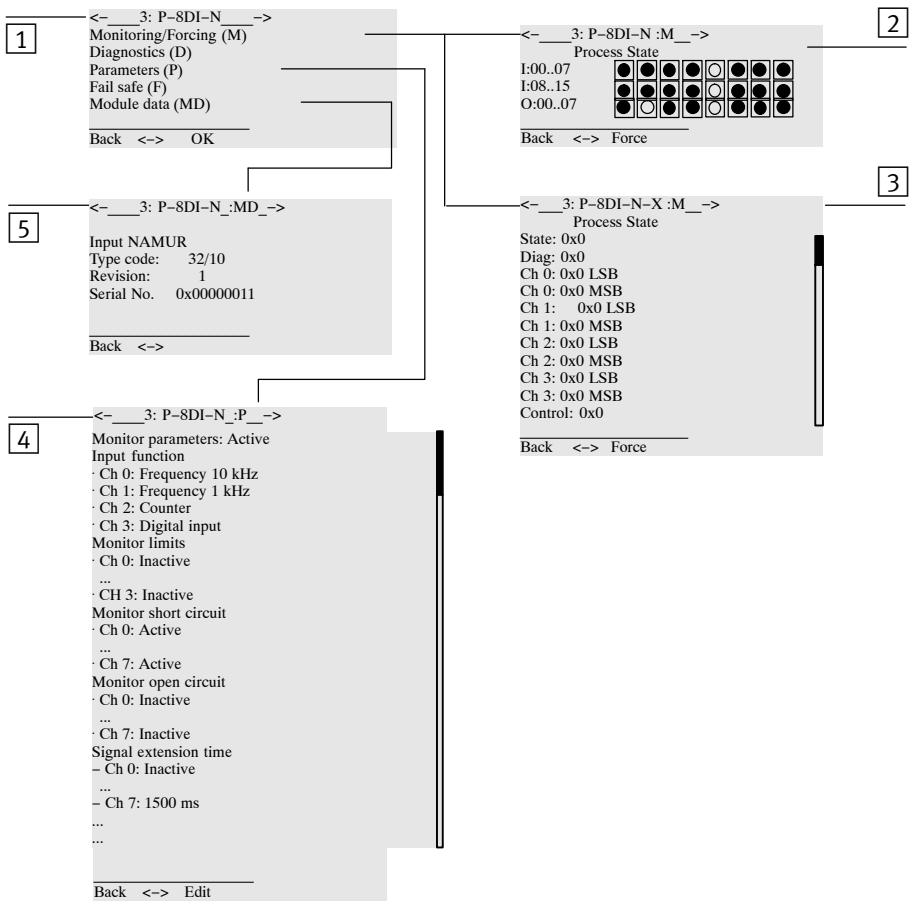
Fig. 18 Spezielle Darstellungen für CPX-P-8DE-N.. am Handheld – Beispiel
