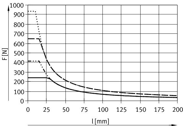
DFM-32 ... 63-KF, Hub bis 50 mm
