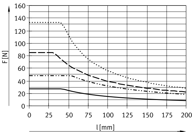
DFM-12 ... 25-KF, Hub bis 30 mm
