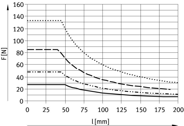
DFM-12 ... 25-GF, Hub bis 30 mm
